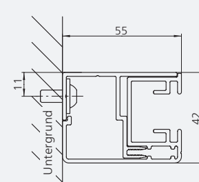
Laibungsmontage
