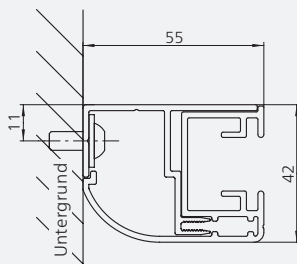
Laibungsmontage
