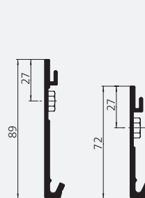
Wandkonsolen für 75 und 92 mm Kassetten
