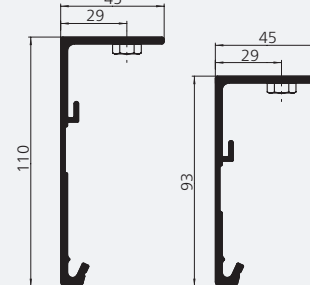
Deckenkonsolen für 75 und 92 mm Kassetten
