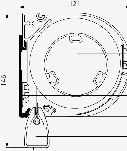
Führungsschiene, rund
